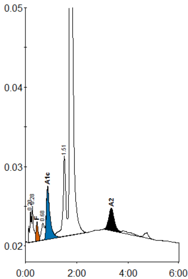
Peak table - ID: 11164984
